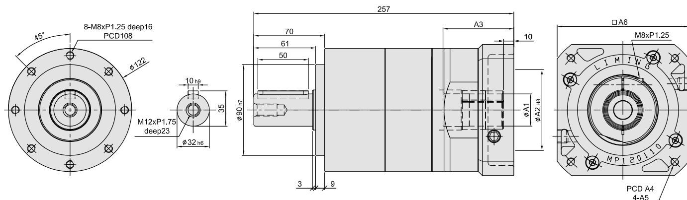
Wymiary kołnierza wejściowego / Dimension of Input Flange
