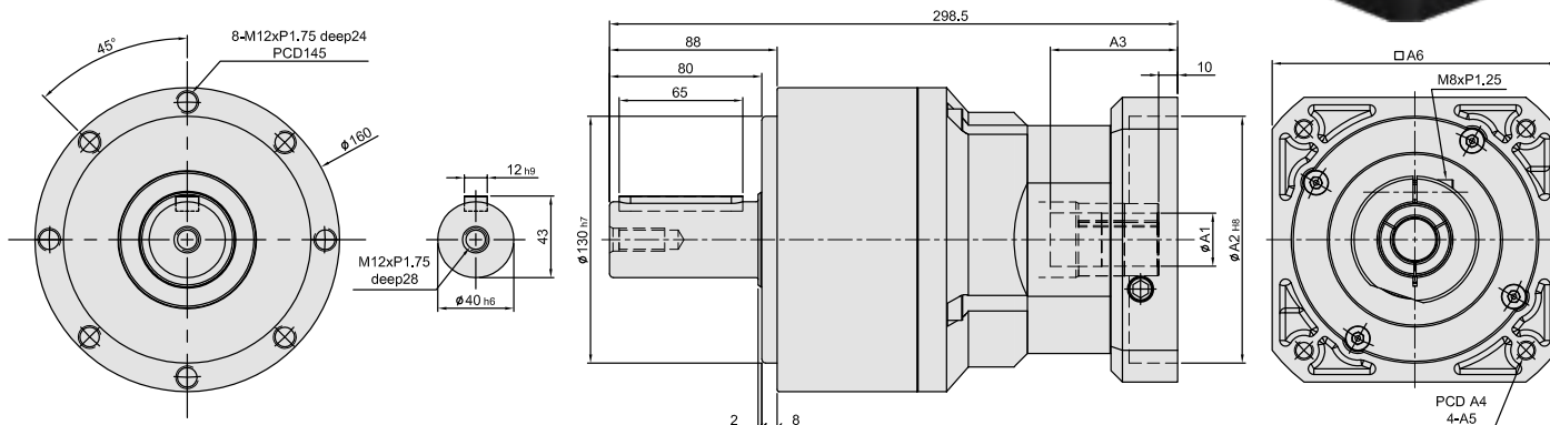
Wymiary kołnierza wejściowego / Dimension of Input Flange
