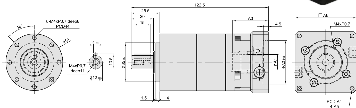
Wymiary kołnierza wejściowego / Dimension of Input Flange
