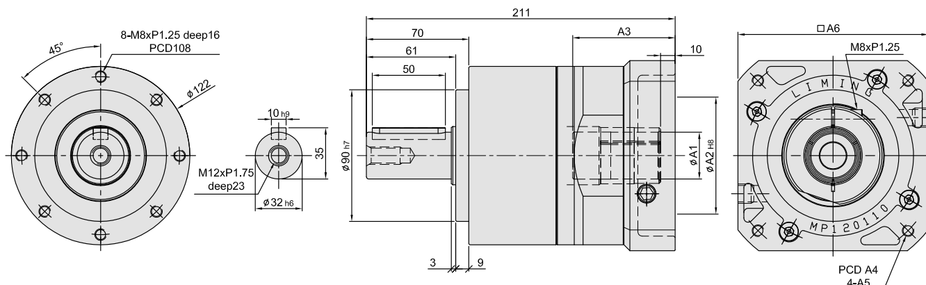
Wymiary kołnierza wejściowego / Dimension of Input Flange
